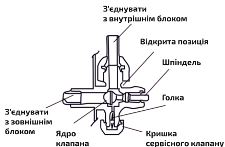
СХЕМА ЧОТИРЬОХ-ХОДОВОГО КЛАПАНА
